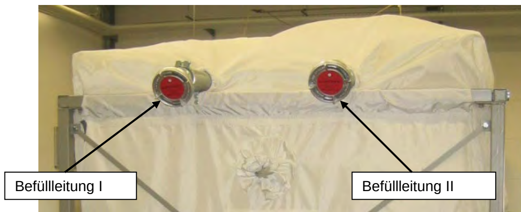
Pelletsilo silos24 mit zwei Befüllstutzen
